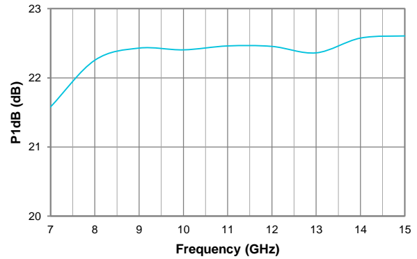
P1dB
